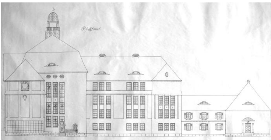
Bauzeichnung der rückseitigen Ansicht der Lessingschule (Stadtarchiv Kamenz)
