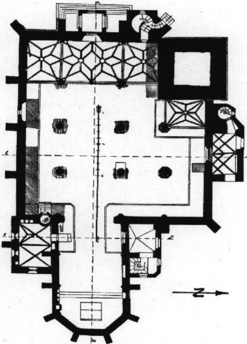
Erdgeschossgrundriss der Marienkirche.
